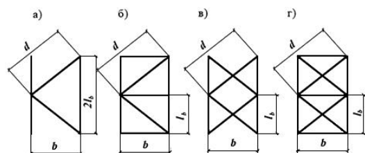
Рисунок 3 - Схемы решеток сквозных стержней
