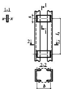
Рисунок 4 - Сквозной стержень с планками
