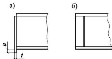
Рисунок 11 - Схема опорного ребра жесткости
