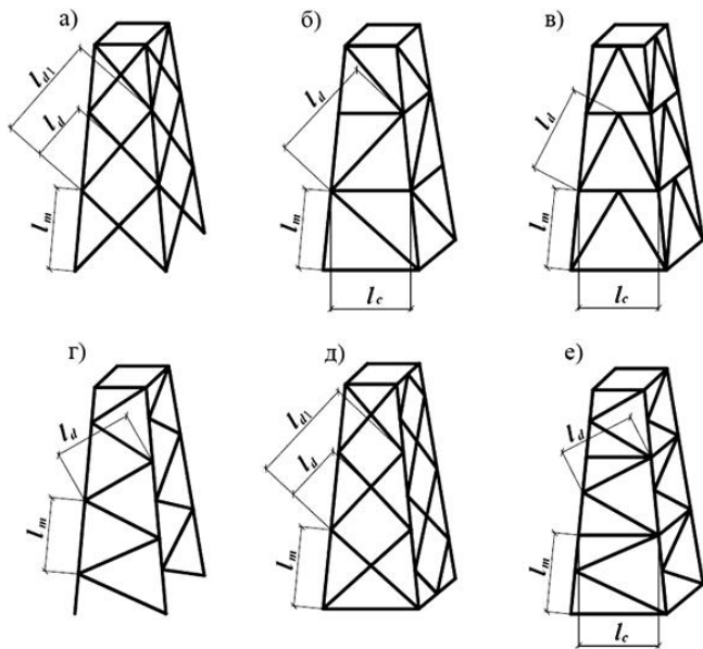
Рисунок 15 - Схемы пространственных решетчатых конструкций
