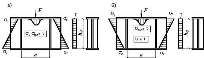
Рисунок 8 - Схема участка балки, укрепленной поперечными ребрами жесткости
