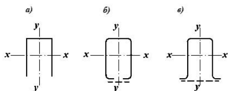
Рисунок 2 - П-образные сечения элементов
