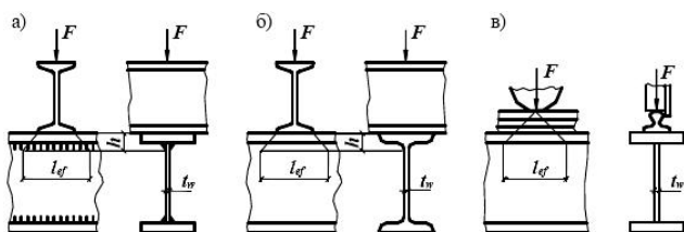
Рисунок 6 - Схемы распределения сосредоточенной нагрузки на стенку балки
